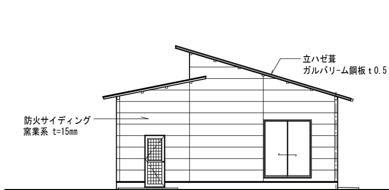
西立面図 1/120
