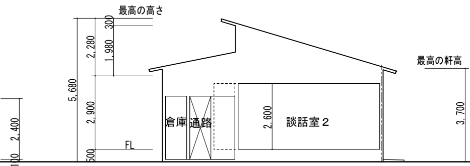
Y方向断面図 1/120
