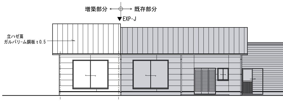
南立面図 1/120
