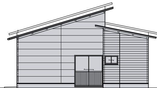
東立面図 1/120
