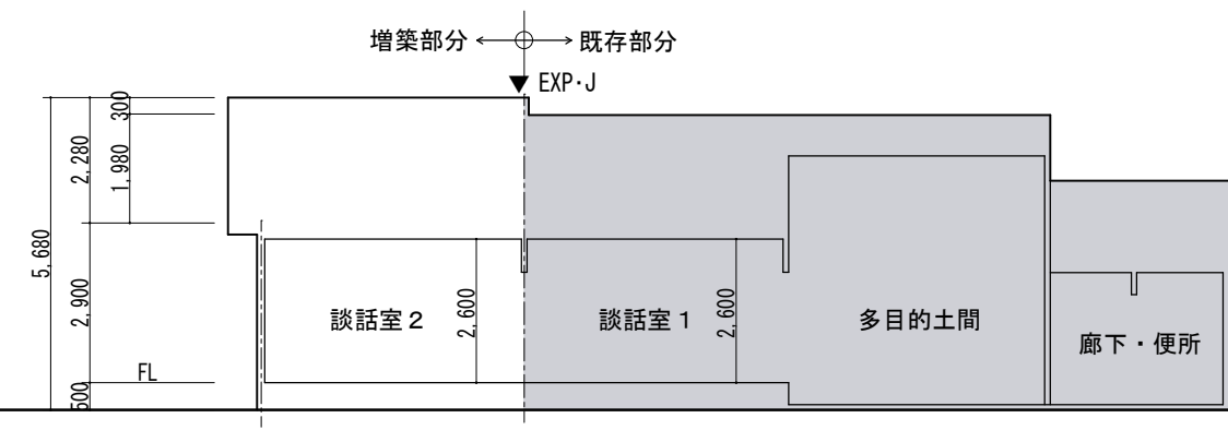
X方向断面図 1/120
